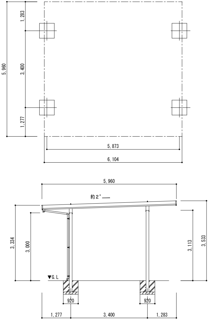
■基礎配置図
